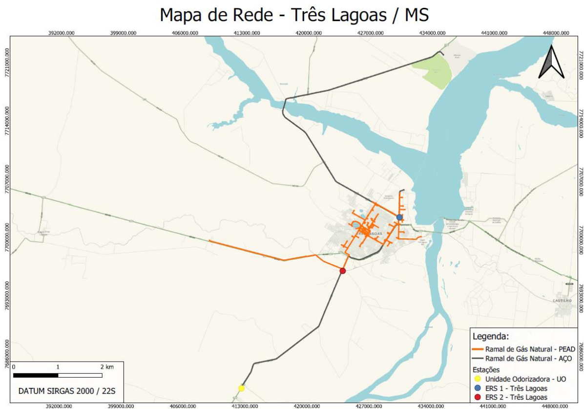
Figura 1. Traçado geral da rede de distribuição de gás natural de Três Lagoas/MS.
